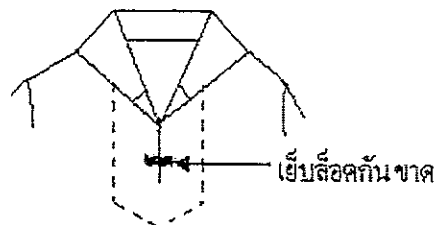
รูปที่ 2 ตัวอย่างการเย็บล็อกคั่นขาดปกเสื้อแบบทหารเรือ
