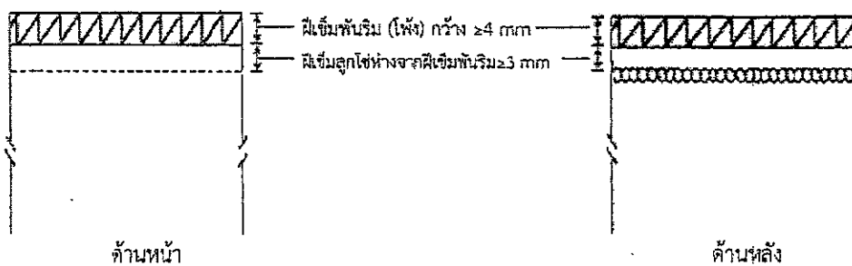
รูปที่ 1 การเย็บผีเข็มพันริมและผีเข็มลูกโซ่
