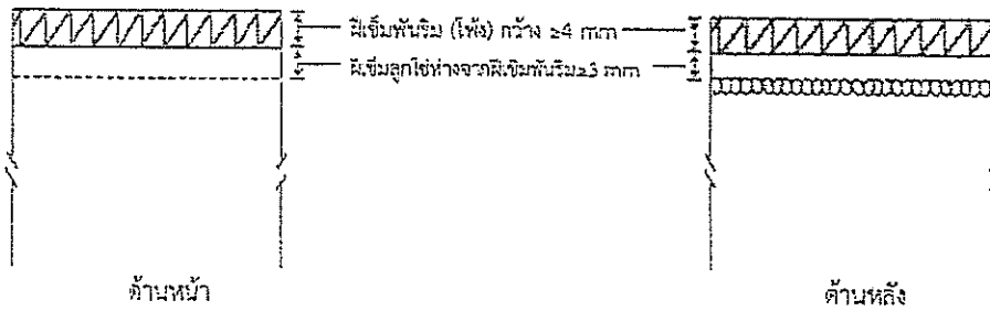
รูปที่ 1 การเย็บฝีมั้ริมและฝีมั้ลูกโซ่
